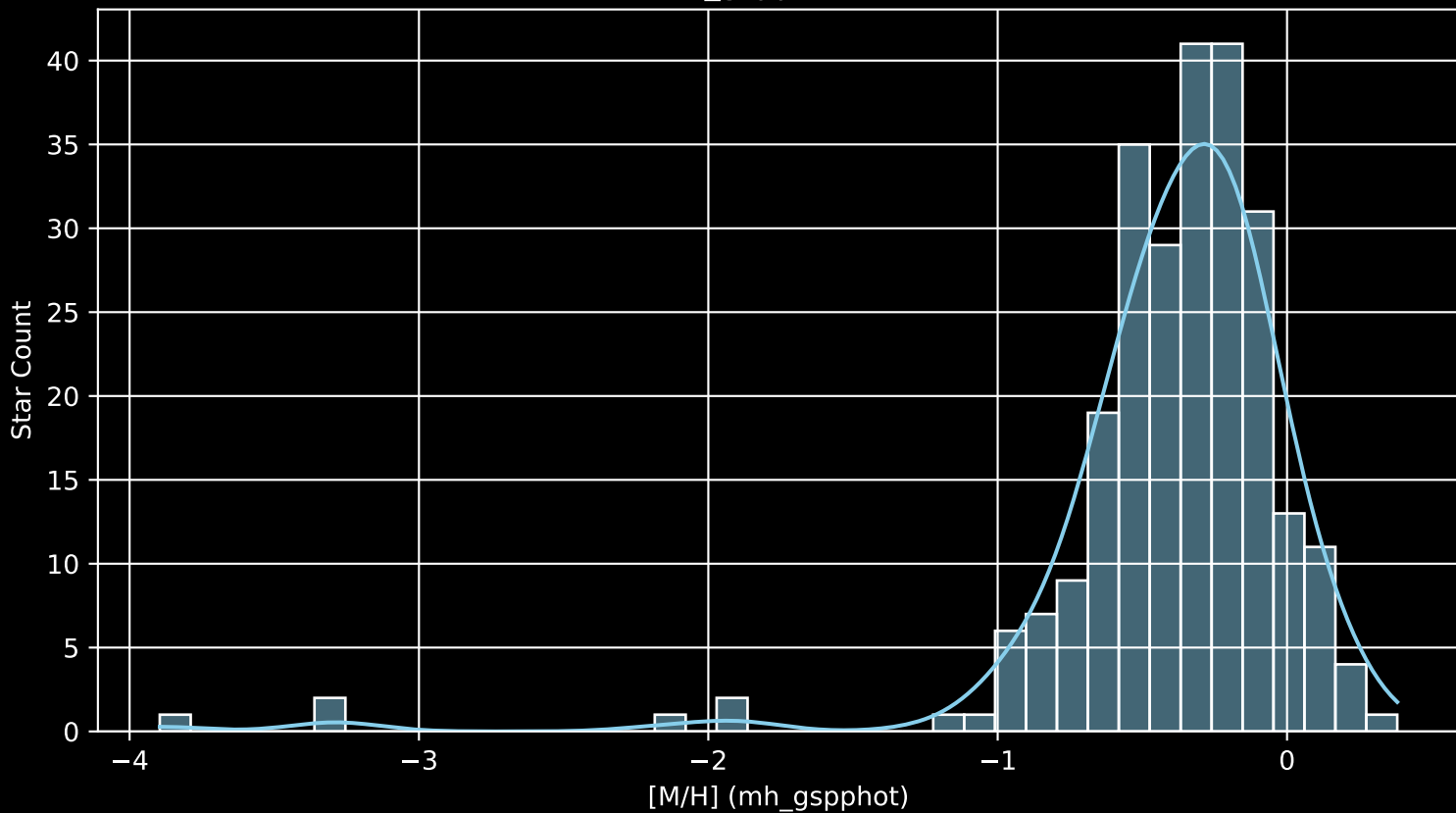
GALAH DR4 Field: [8754] [M/H] (mh_gspphot) (n= 255)
