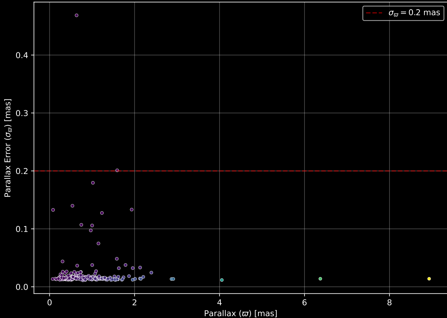
GALAH DR4 Field: [8754] Parallax Quality (n= 256)
