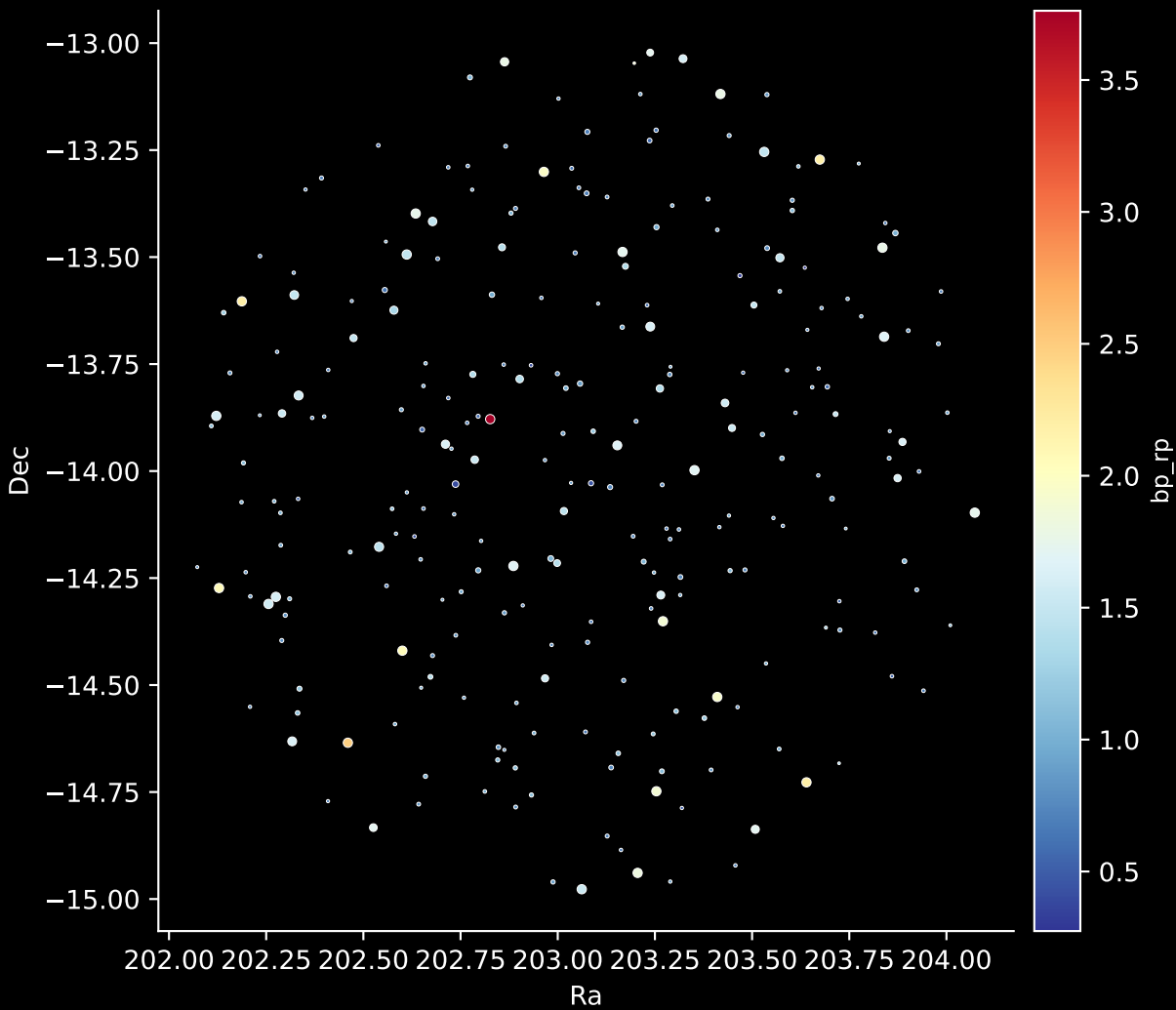
GALAH DR4 Field: [8754] Stars: 256
