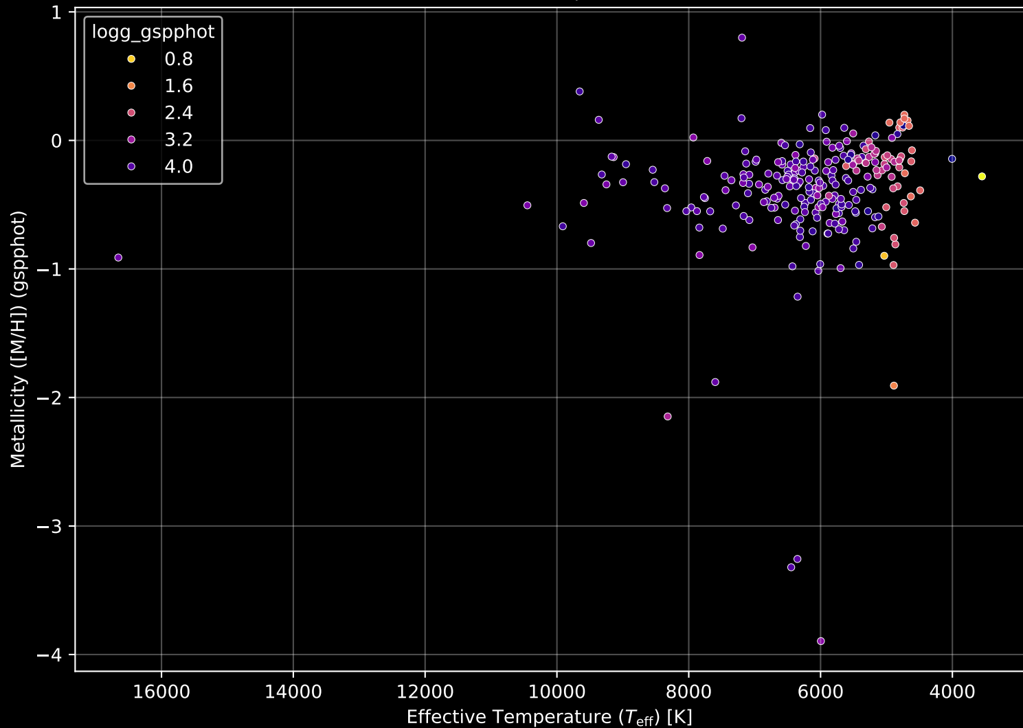
GALAH DR4 Field: [8754] Stellar Population Parameters (n= 256)
